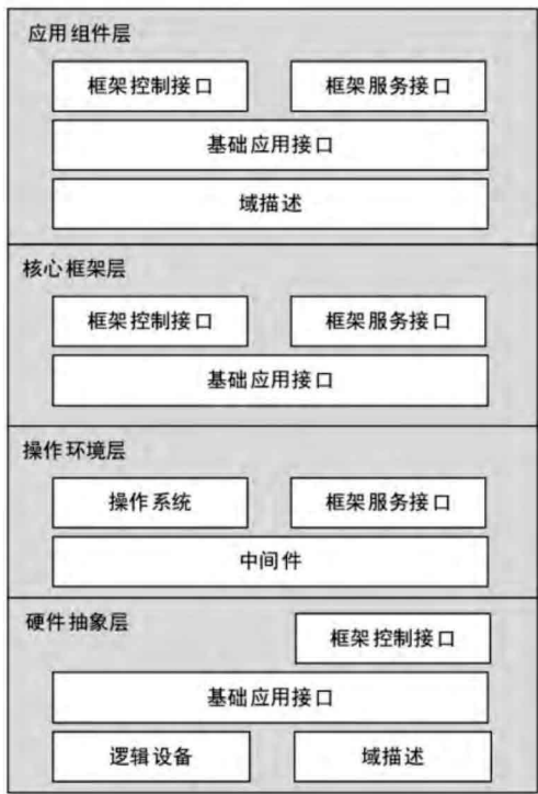
图3 SCA 软件架构
