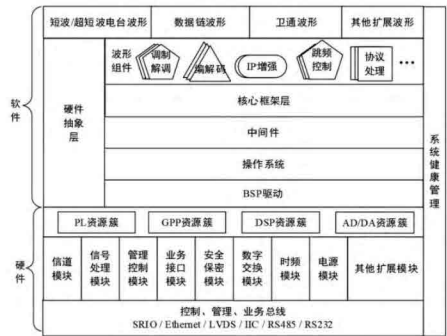
图1 软件无线电通信平台软硬件总体架构
