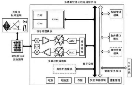
图2 多体制软件无线电通信平台硬件架构
