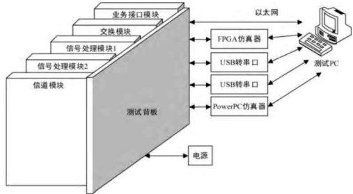
图5 测试验证平台
