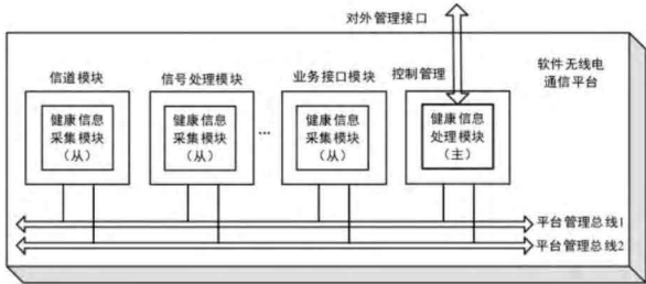
图4 软件无线电通信平台健康管理系统
